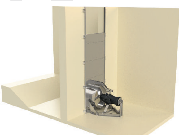
Zirkulationsrahmen mit U-Schienen Circulation Frame with U Rails
