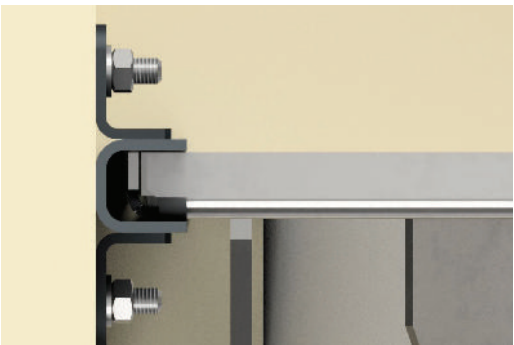
Verbindungsdetails von Umlaufrahmen mit U- und Z-Schienen Connection details of circulation frames with U and Z rails
