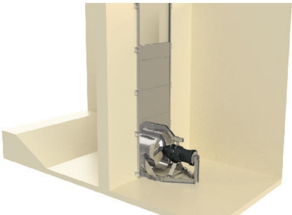
Zirkulationsrahmen mit Z-Schienen Circulation Frame with Z Rails
