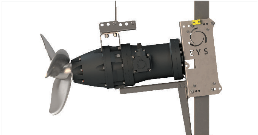
Einbau bei -7° zur Aktivierung der am Boden abgesetzten Feststoffe Installation with -7° to activate settled solids at the bottom
