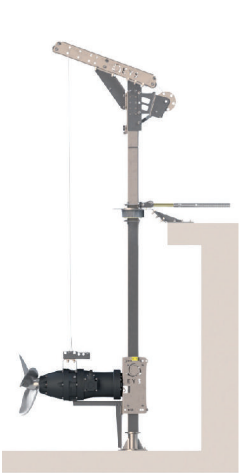
Standard- Positionierung Standart positioning
