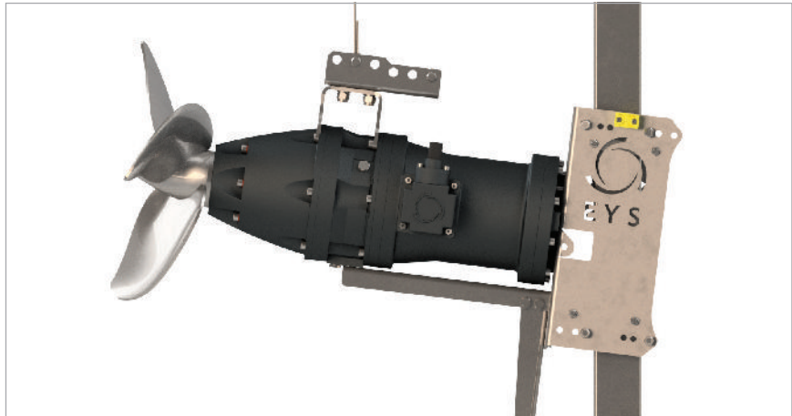
Einbau mit +7° zum Brechen fester Schwimmdecken auf der Oberseite Installation with +7° to break solid plug on top
