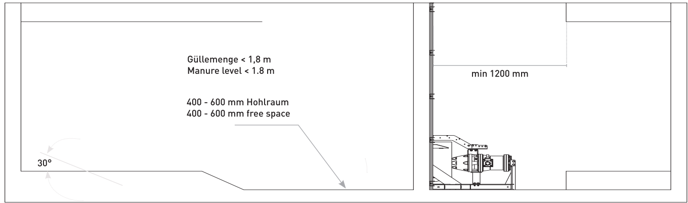
Positionierung von Tauchmotorrührwerken in Slalomgruben und in Gängen Positioning of submersible mixers in slalom type pits and in corridors
