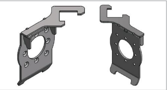
Fangflansch mit Gleitführung für DP Serie Tauchmotor Pumpen Sliding flange for DP series submersible pumps
